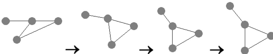
Abbildung 2: Ablauf des Spring-Embedders
