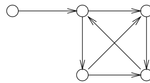
gerichteter Graph
